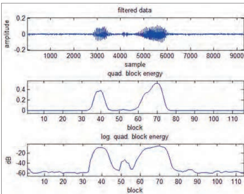
Bild 5: Amplitude und Energie- verläufe des Wortes „rückwärts“
