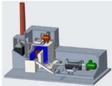
Biomasse- Kraftwerk (CAD- Modell)
