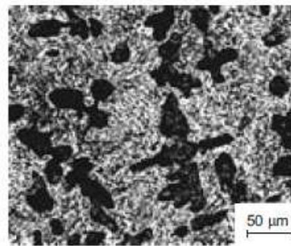
b) PbSn50
