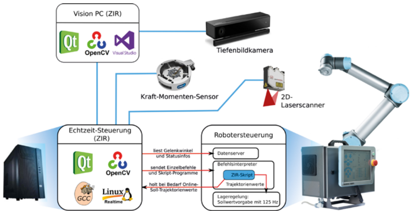
Technologische Übersicht für die Mensch-Roboter-Interaktion am ZIR
